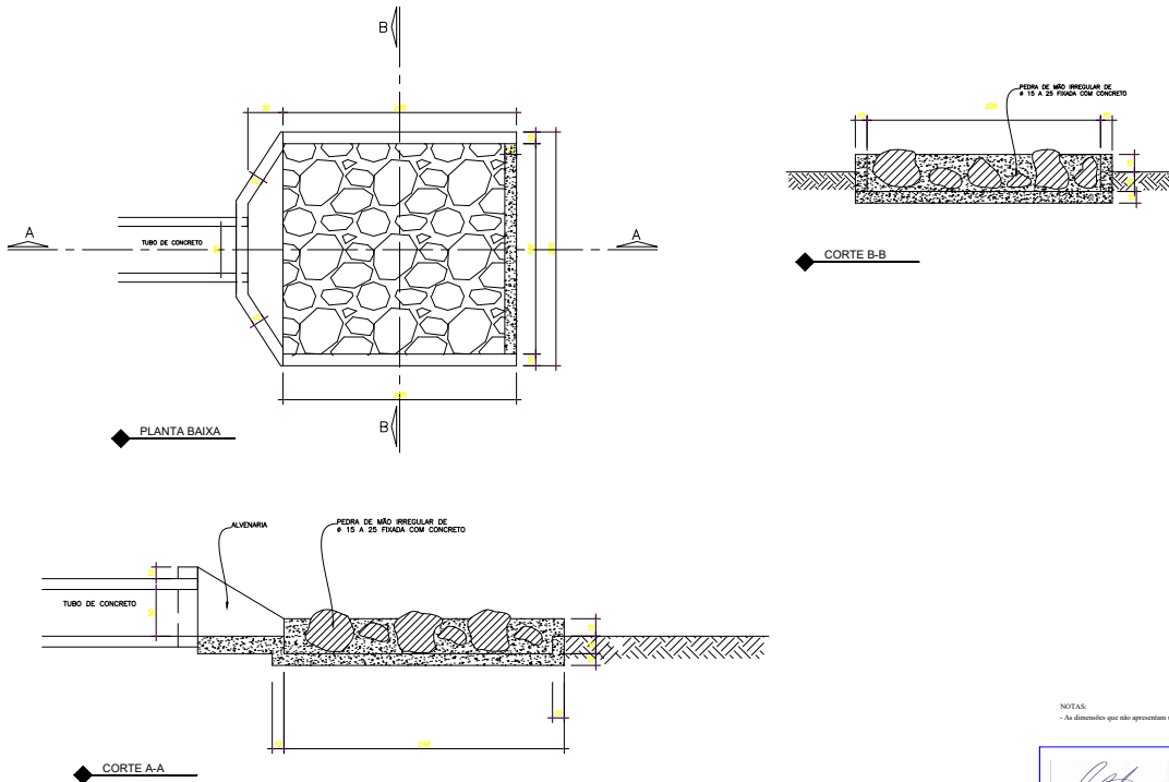
DETALHE - DISSIPADOR DE ENERGIA
